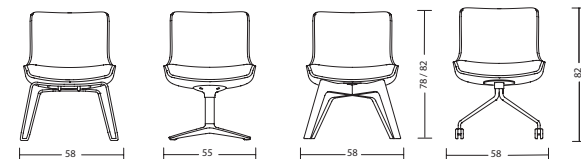
woo56 + 3246 / 3231 / 3206 / 3226 ohne Armlehne without armrest 7 kg
