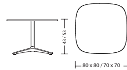
woo25 Gewicht Weight 11 kg / 12 kg
